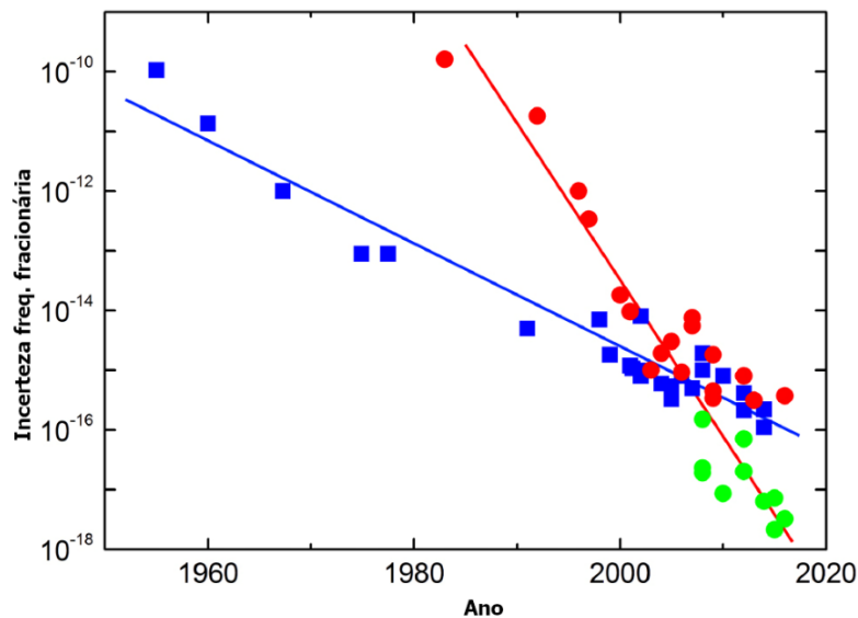
Figura 1 - Evolução da incerteza fracionária. Quadrados azuis representam padrões primários de céσιο. Círculos vermelhos representam padrões de frequência óptica comparados diretamente com relógios atômicos de céσιο. Círculos verdes representam incertezas estimadas publicadas de relógios ópticos. Linhas azul e vermelha mostram tendência dos padrões primários e ópticos, respectivamente. Adaptado de [2].
