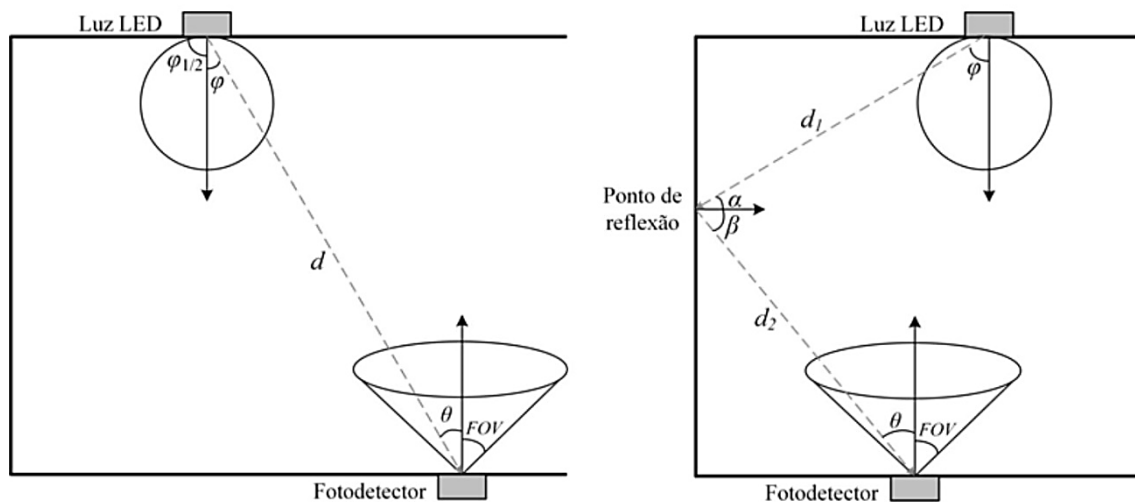
Figura 1 - Comunicação por LED: (a) linha de visada e (b) caminho indireto
