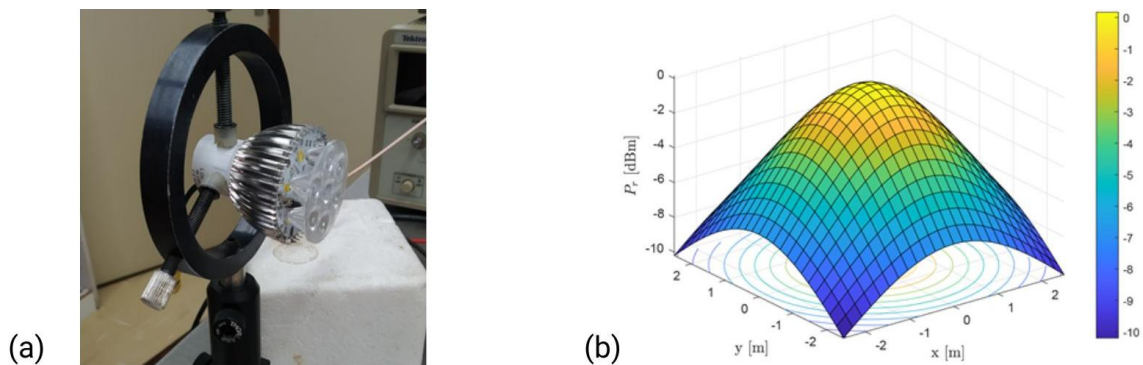
Figura 2 - (a) Luminária LED; (b) distribuição de potência em uma superfície.
