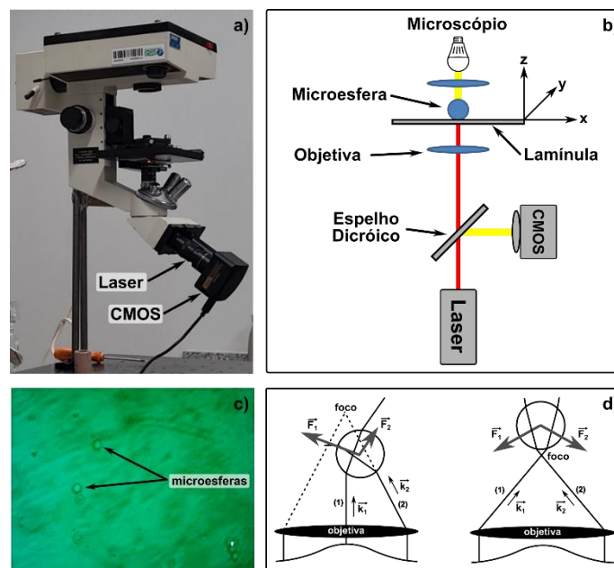
Figura 2 - Montagem do microscópio de objetiva invertida para pinça óptica: a) Fotografia da montagem; b) Esquema da configuração da pinça óptica; c) Imagem capturada pela câmera CMOS das microesferas focalizadas; d) Esquema ilustrando as forças atuantes na microesfera na região do foco do laser.
