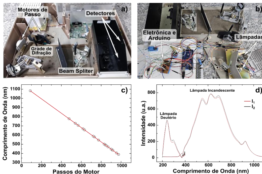
Figura 3 - Montagem do espectrofotômetro: a) Fotografia da parte interna; b) Fotografia da parte interna com eletrônica e Arduino integrados; c) Ajuste linear para a calibração do comprimento de onda dos picos de emissão das lâmpadas; d) Espectro das lâmpadas de vapor de deutério e incandescente após a calibração.
