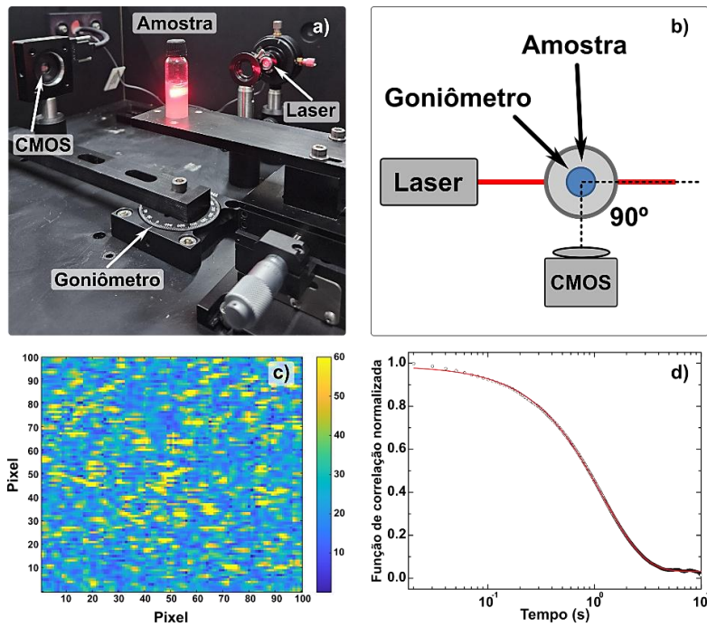
Figura 4 - Montagem do espalhamento de luz dinâmico (DLS): a) Fotografia do setup óptico montado dentro de uma caixa para evitar interferência de luz externa; b) Esquema ilustrativo da montagem do setup óptico; c) Exemplo de uma imagem de espalhamento Speckle obtida pela câmera CMOS; d) Curva de autocorrelação temporal normalizada da intensidade da luz espalhada ajustada com uma função exponencial simples.
