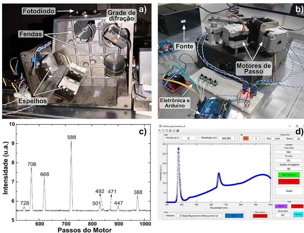
Figura 1 - Montagem do espectrômetro: a) Vista interna, destacando os principais componentes; b) Vista externa mostrando a estrutura física e disposição dos elementos; c) Espectro da lâmpada de hélio em relação aos passos do motor, com valores de comprimento de onda em nanômetros; d) Interface gráfica desenvolvida no MATLAB (GUIDE) para operação do espectrômetro.
